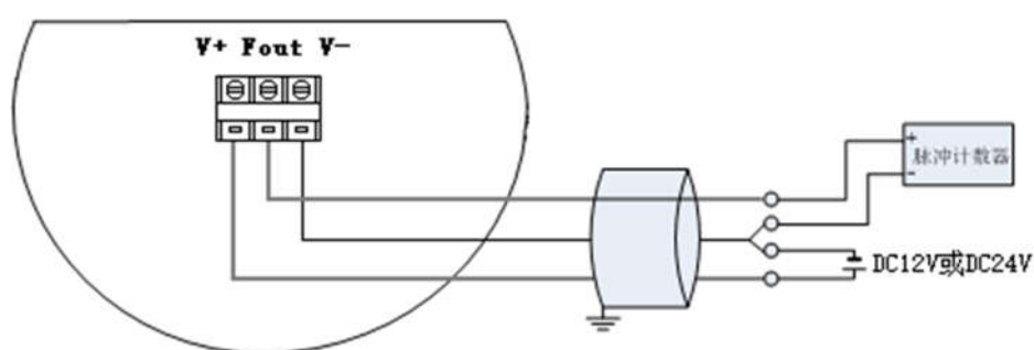
VM 无显示型信号处理电路（脉冲型）
