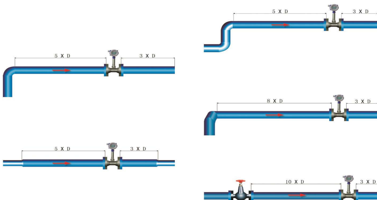
宽量程型涡街流量计上下游直管段预留尺寸图
