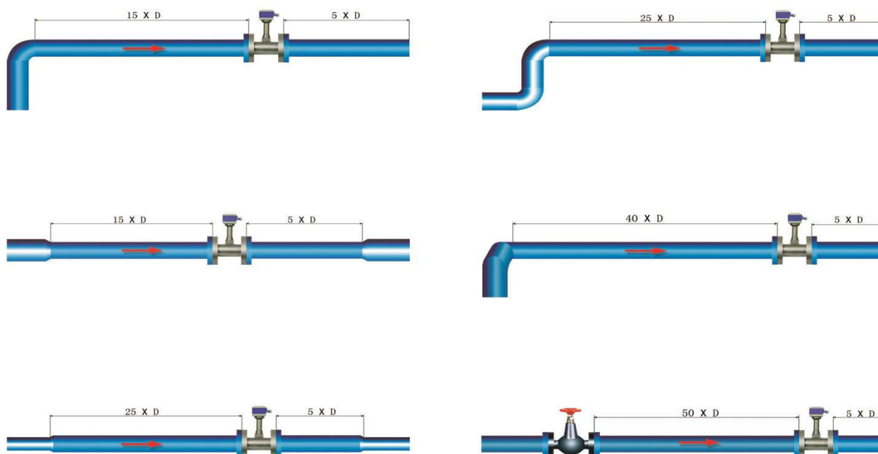
标准型涡街流量计上下游直管段预留尺寸图
